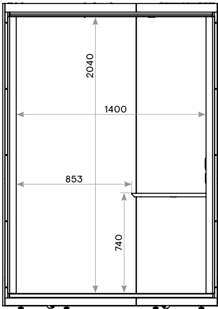
Vorderansicht
