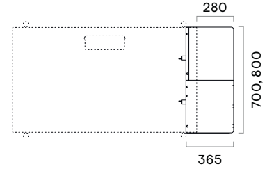
Draufsicht auf seitliche Metallschubladen in Kombination mit Schreibtischen
