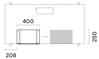
Draufsicht auf die untergebaute Metallschubladen in Kombination mit Schreibtischen
