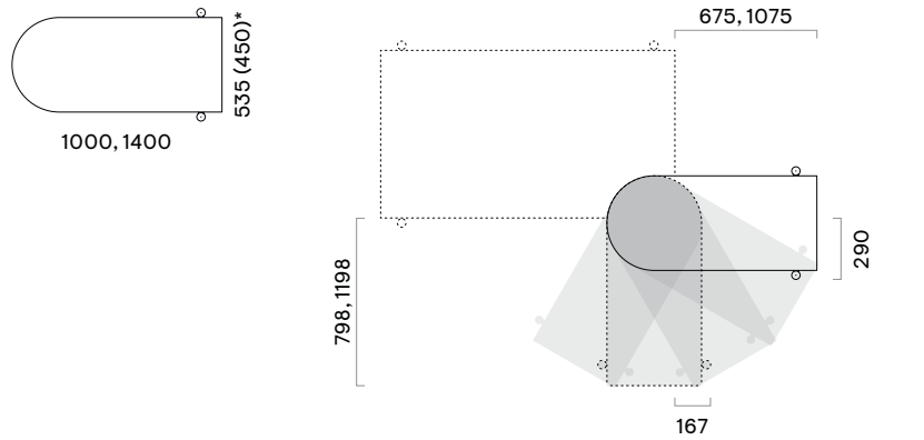
Draufsicht auf den Anstellisch in Kombination mit dem Schreibtisch
